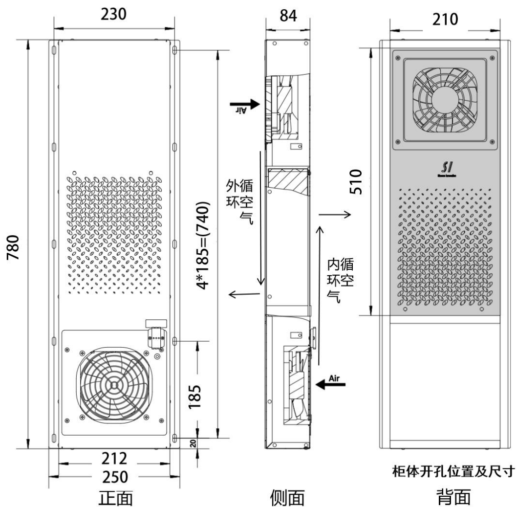
产品尺寸图：
